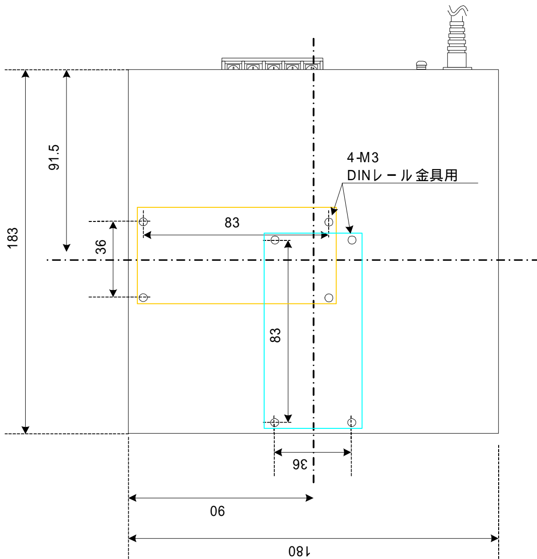
【 Enet-485/ AC DINレール取付金具穴位置寸法図】
