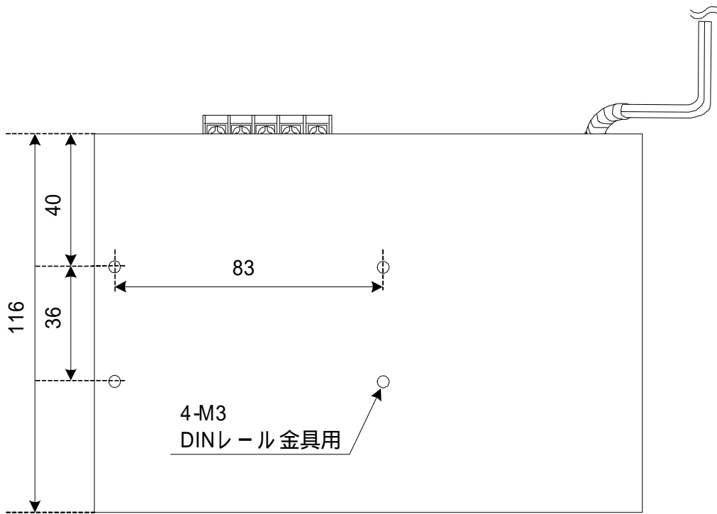
【 DINレール取付金具穴位置寸法図】
