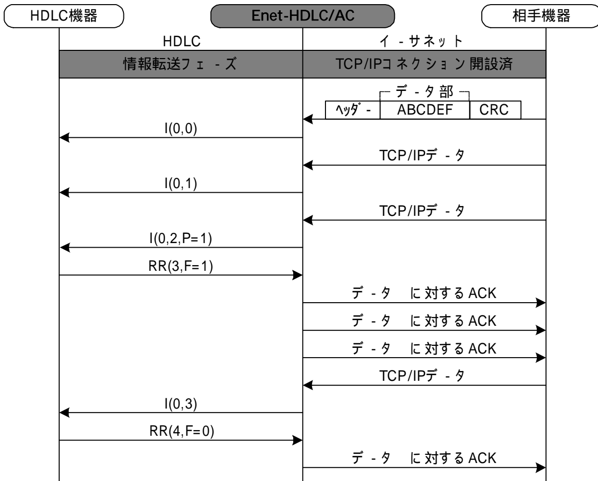
Enet-HDLC/AC プログラムモード設定 OC=3の場合
