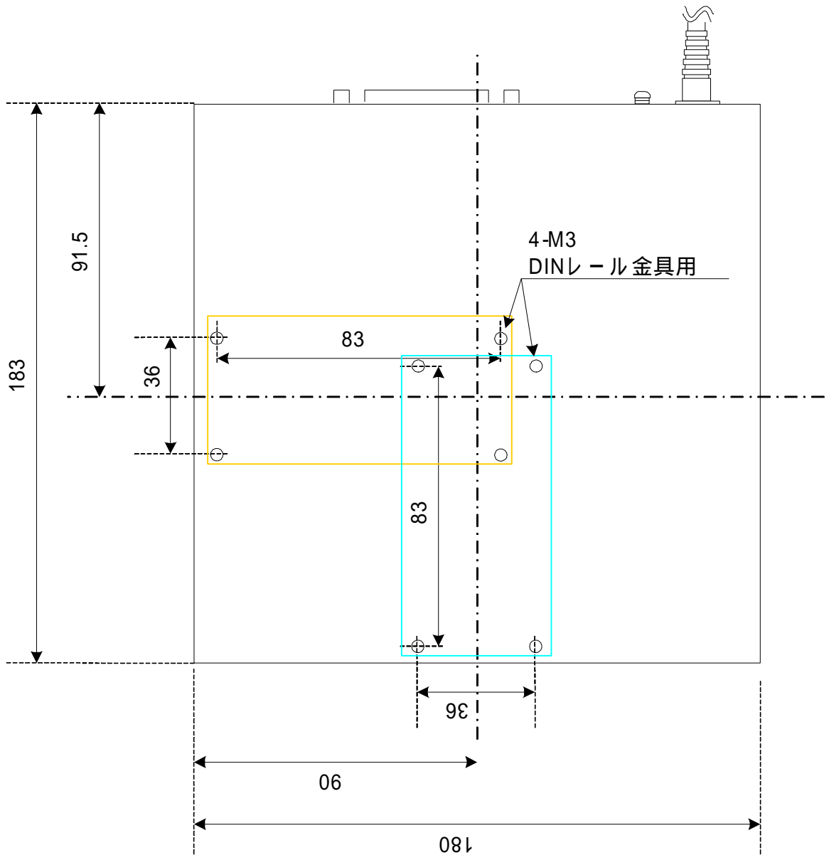
【 Enet-HDLC/ AC DINレール取付金具穴位置寸法図】
